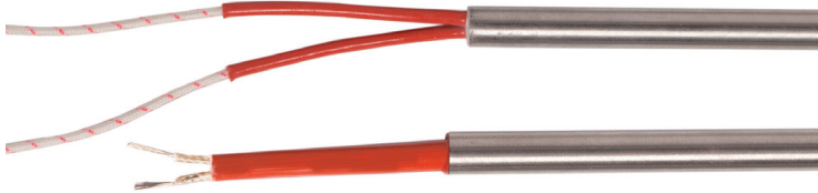
Kabelschutz mit Glasseiden-Silikonschlauch (einzeln pro Kabel oder gemeinsam)
